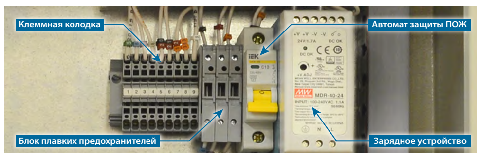
Устройство шкафа АВР
